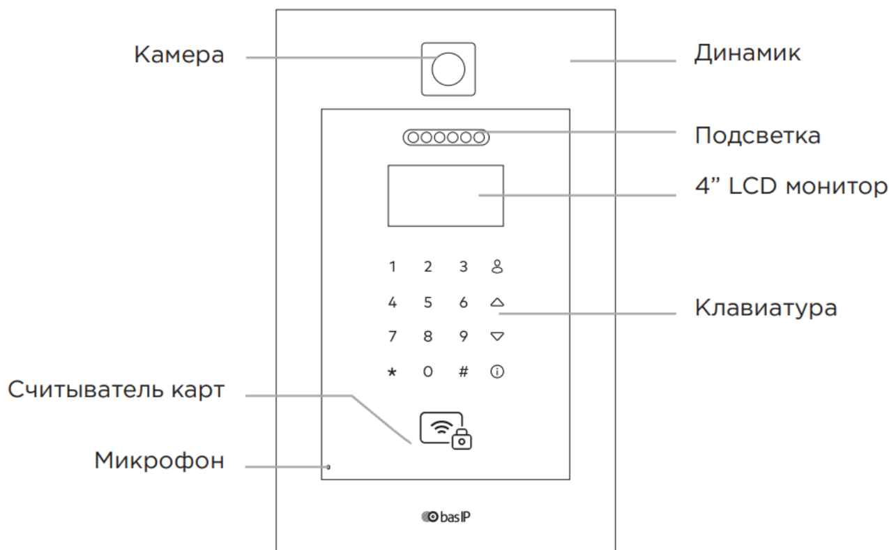
Рис. 5. Внешний вид и органы управления блока.
